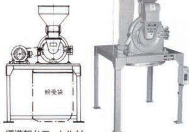
標準架台モートル付
