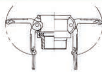
MAX-B PT雌ねじカバー ※この商品のみSUS304製となります。
