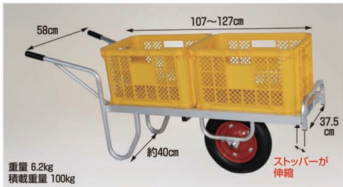
CN-35D エアータイヤ(TR-13×3T) 本体価格 20,400円(税別) ※CN-35Dは在庫が終わり次第ハイパンです。 (変更) (送料) 4台で元払い(離島は別途)(1台梱包)
