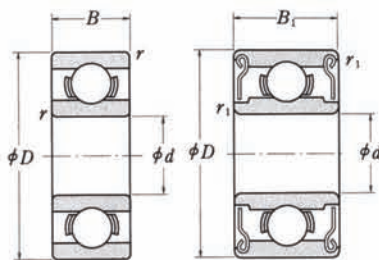
シールド形 ZZ・ZZ1
