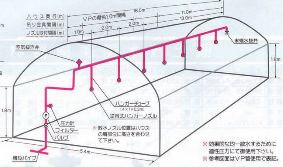
配管設置例 (5.4m×18.0m)=30坪
