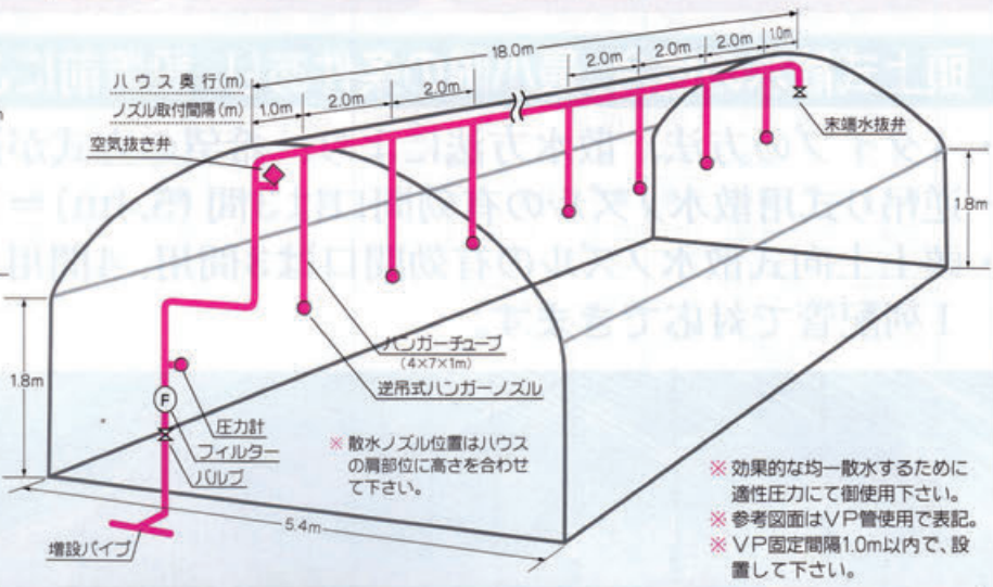
D3-1タイプ 頭上逆吊り式散水法・関連部品明細 ハウス面積(5.4m×18.0m)=97.2㎡
