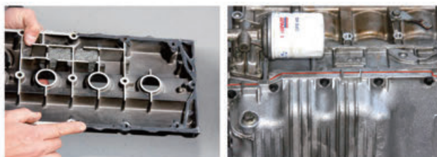
エンジンブロックの合わせ面 オイルパンの合わせ面
