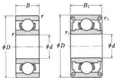
シールド形 ZZ・ZZ1
